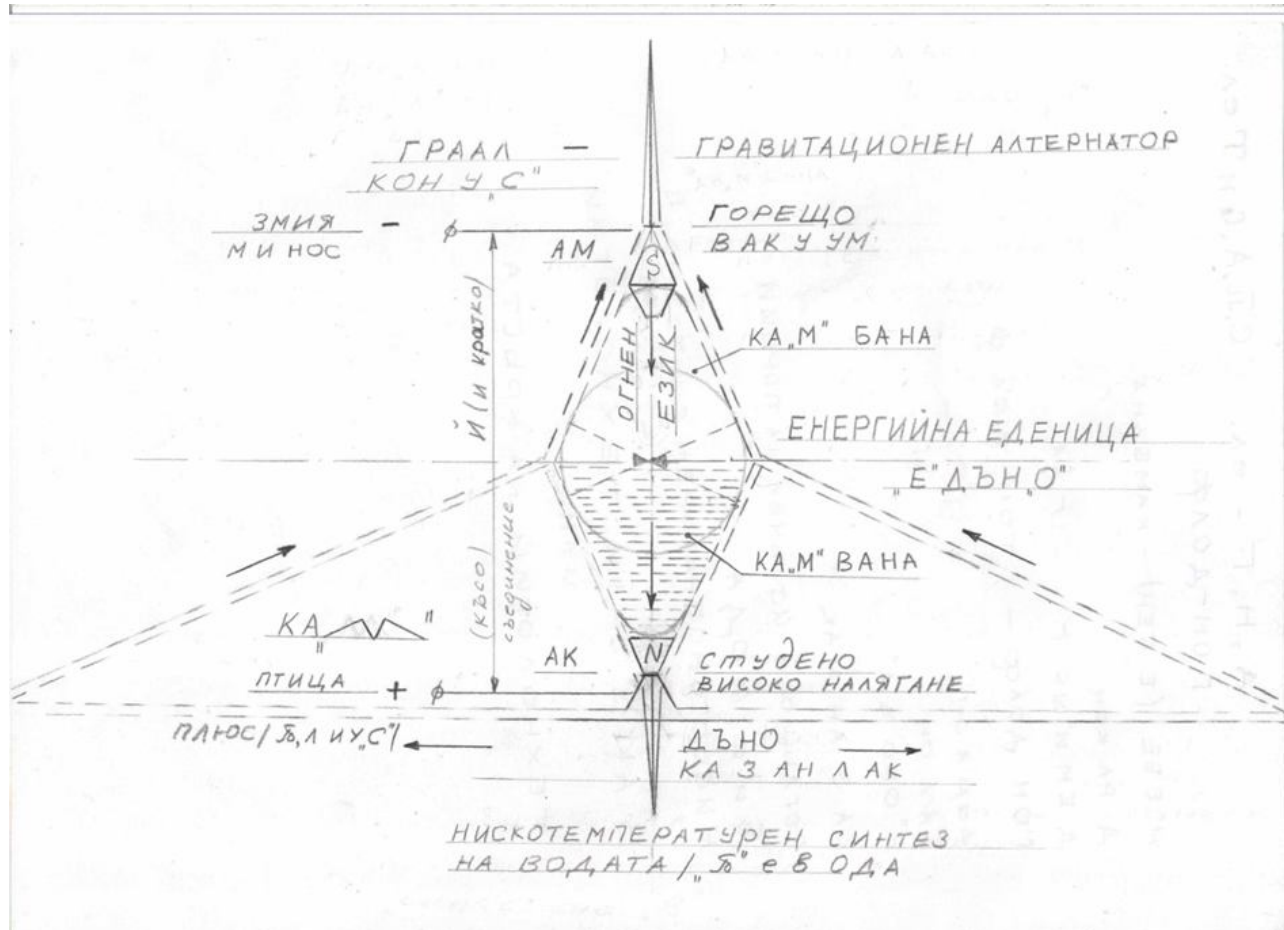
Фиг. 2 Форма: ВАНА Г. Слънчево- гравитационен потенциал
